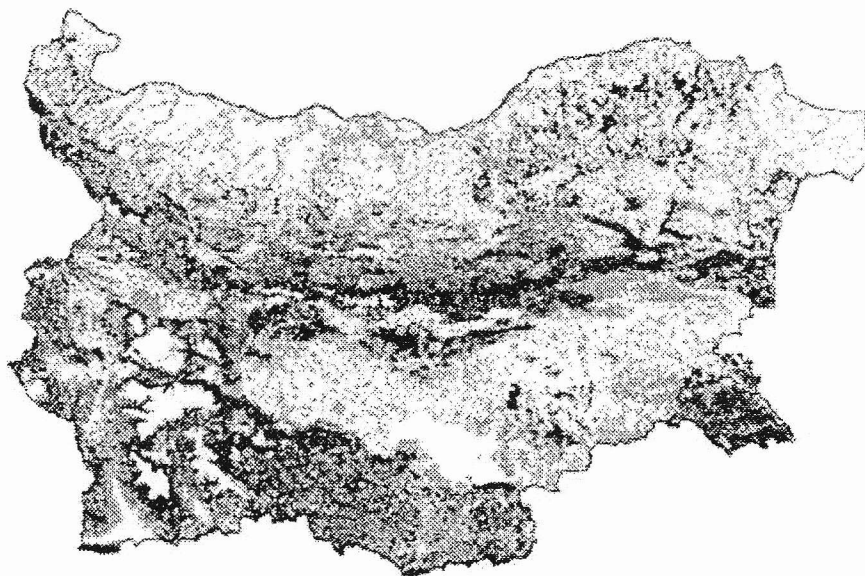
Карта 33. Podarcis muralis
